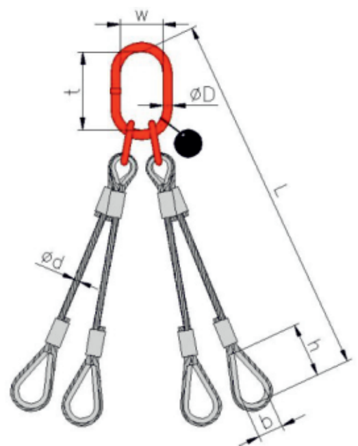
oceľové lano OKO-4OKA lisované s očnicami
