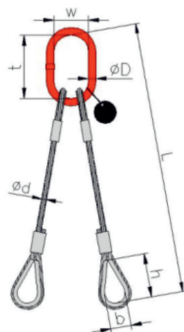
ocel'ové lano OKO-2OKA lisované s očnicami
