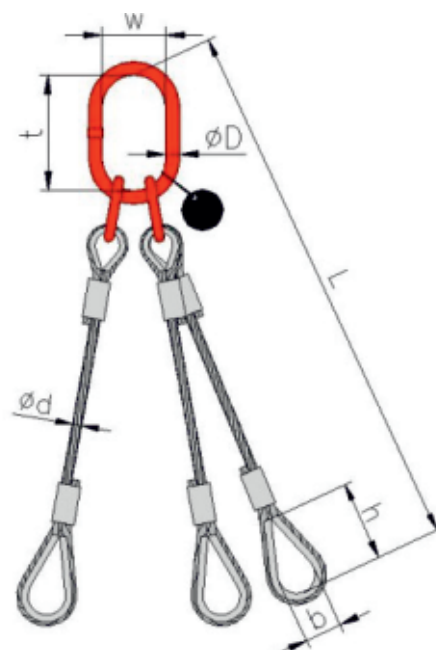
oceľové lano OKO-3OKA lisované s očnicami
