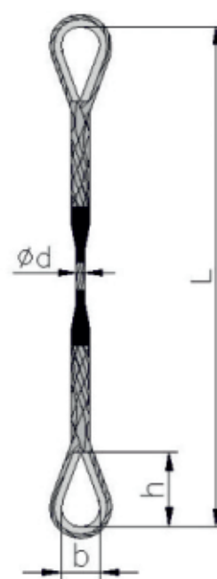
ocel'ové lano OKO-OKO zapletané s očnicami
