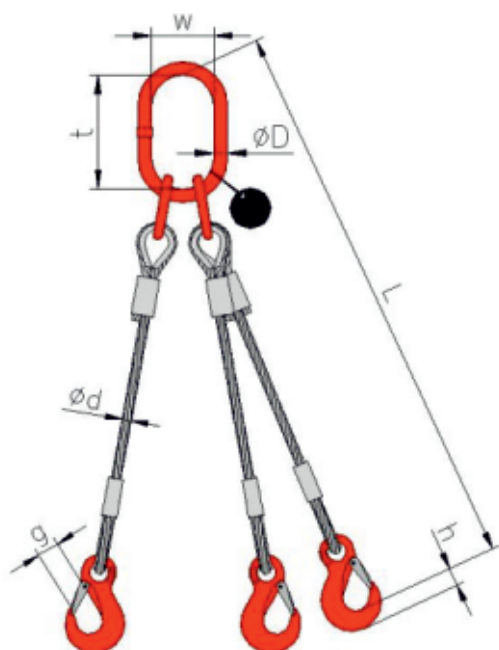
oceľové lano OKO-3HAK lisované
