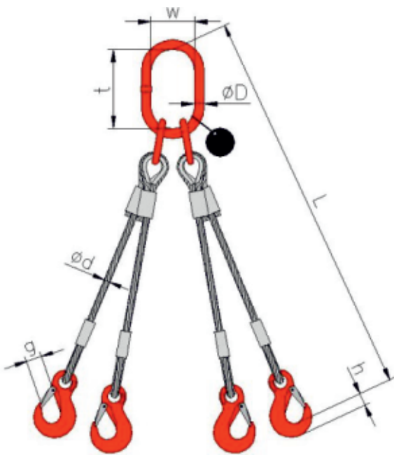
oceľové lano OKO-4HAK lisované
