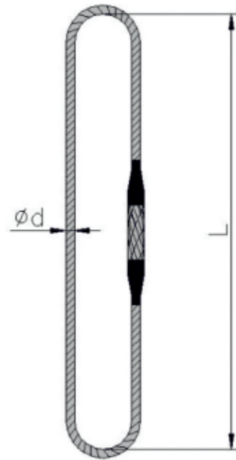
oceľové lano nekonečné zapletané
