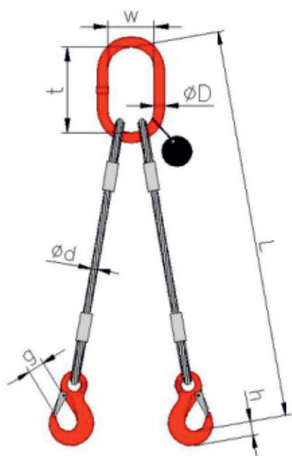
ocel'ové lano OKO-2HAK lisované
