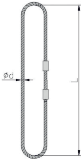
oceľové lano nekonečné lisované
